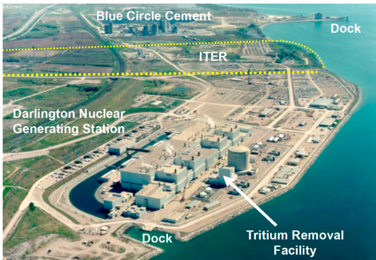
Fot. 2. Zdjęcie proponowanej instalacji ITER pomiędzy elektrownią jądrową Darlington (4 x 930 MW brutto) i przyległą cementownią (w obrębie żółtej linii przerywanej). Propozycja wg dokumentów złożonych kiedyś w urzędzie regulacyjnym energii jądrowej CNSC.
