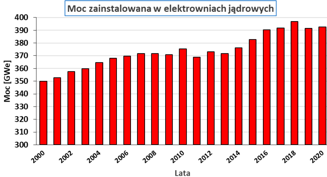
Rys. 1. Zmiana zainstalowanej mocy w elektrowniach jądrowych na świecie w latach 2000-2020
