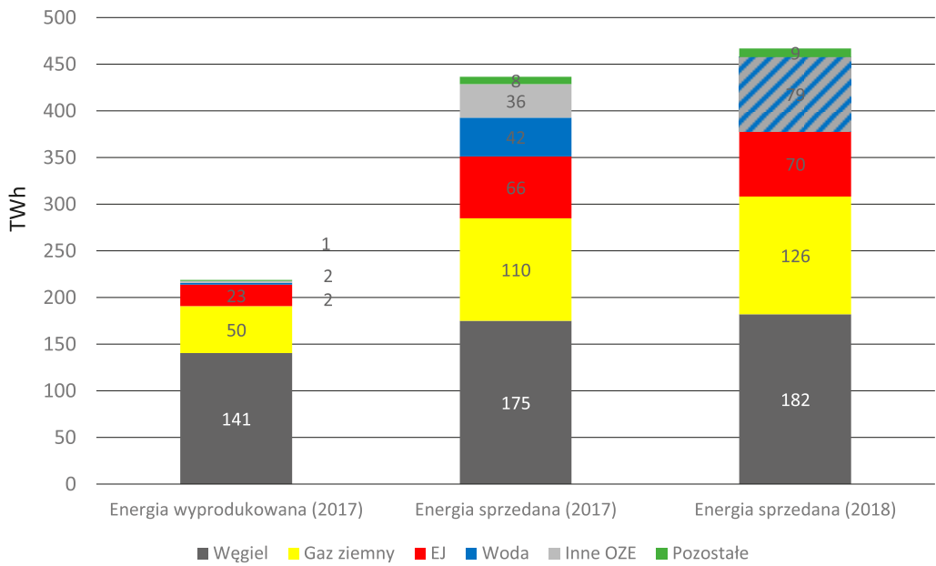
Rys. 4. Struktura energii elektrycznej wyprodukowanej i sprzedanej w 2017 r. i 2018 r. przez spółdzielnie energetyczne w USA Fig. 4. A structure of electricity generated and sold by American co-ops in 2017 and 2018. Źródło: opracowanie własne na podstawie: America's Electric Cooperatives [https://www.electric.coop/wp-content/uploads/2020/06/Coop_FactsAndFigures_June2020.pdf] (dostęp: 2020-11-19); Electric industry generation, capacity, and market outlook, J. Goodenberry, A. Hamilton, L. Khair, M. Leitman, A. Brown, NRECA, 2019, s. 3. [https://www.cooperative.com/programs-services/bts/resource-adequacy-markets/Documents/ram_outlook_report.pdf] (dostęp: 2020-11-19)
