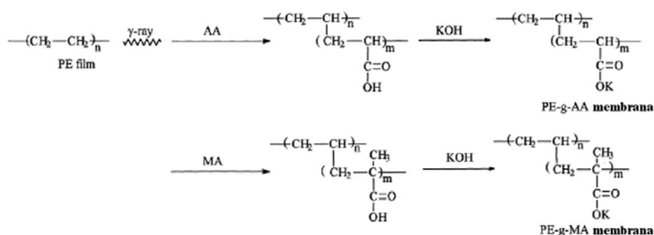
Rys. 7.1. Schemat szczepienia radiacyjnego, szczepienie na folii polietylenowej grup funkcyjnych o zdolnościach jonowymiennych (Reprinted from M.M.Nasef, El-Sayed A.Hegazy, Preparation and application of polar monomers grafting onto non-polar films, Prog. Polym. Sci., 29(6), 499-561, Copyright 2004, with permission from Elsevier).
