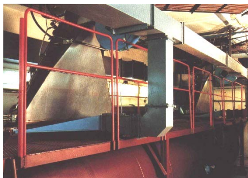
Rys. 9.8. Instalacji pilotowa oczyszczania gazów odlotowych zbudowana w Elektrociepłowni Kawęczyn: A – sterownia; B – widok komory reakcyjnej i układów przemiatania wiązki elektronów
