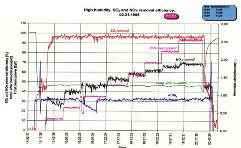
Rys. 9.9. Zależność skuteczności usuwania \text{SO}_2 i \text{NO}_x w zależności od wielkości prądu (mocy) wiązki elektronów
