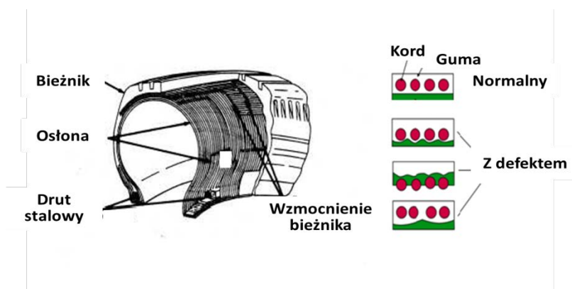
Rys. 5.1. Przekrój poprzeczny opony radialnej oraz możliwe defekty związane z przesunięciem komponentów w procesie wulkanizacji
