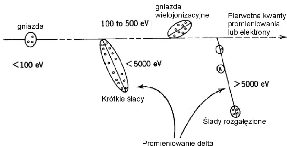
Rys. 2.3. Schemat przedstawiający skutki wywoływane w ośrodku przez promieniowanie jonizujące.
