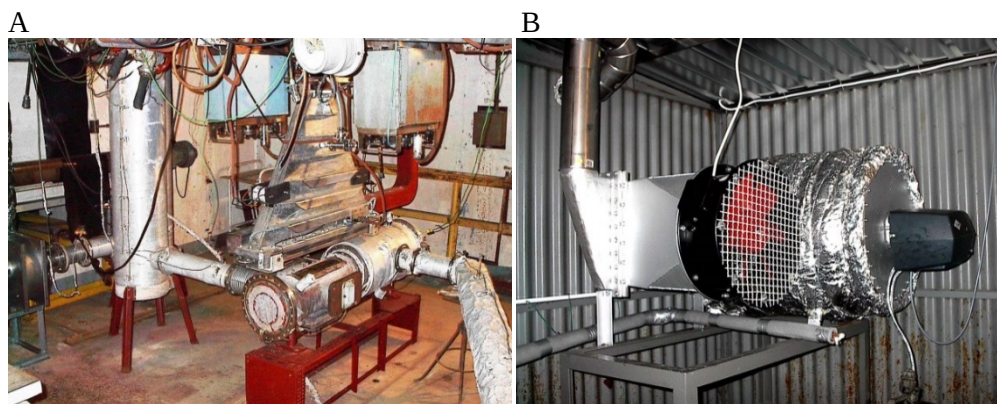
Rys. 9.7. Laboracyjna instalacja zbudowana w Instytucie Chemii i Techniki Jądrowej do prowadzenia badań w zakresie radiacyjnego usuwania zanieczyszczeń z fazy gazowej: A – wyprowadzenie wiązki elektronów oraz komora reakcyjna, B – palnik oleju opałowego jako źródło spalin
