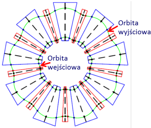
Rys. 3. Schemat funkcjonalny akceleratora typu eFFAG. Orbita wejściowa dla energii iniekcji elektronów 50 keV. Orbita wyjściowa elektronów dla energii 9 MeV (promień <50 cm)
