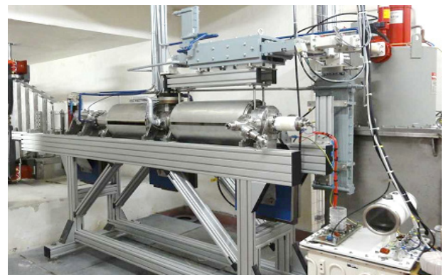
Fot. 8. Widok ogólny liniowego akceleratora elektronów z falą bieżącą zbudowany przez firmę CoRAD z Rosji
