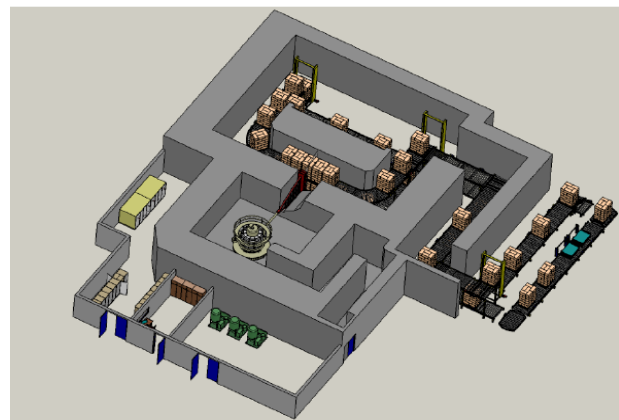
Fot. 6. Makieta instalacji radiacyjnej wykorzystującej akcelerator typu Rhodotron pracujący w reżymie promieniowania hamowania, pracująca w firmie Leoni, Szwajcaria
