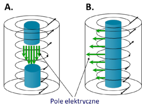
Rys. 1. Konstrukcja rezonatora przyspieszającego wiązkę elektronów: A – z jednym przejściem wiązki przez strefę przyspieszania (akcelerator typu ILU); B – z wieloma przejściami przez strefę przyspieszania (akcelerator typu Rhodotron)
